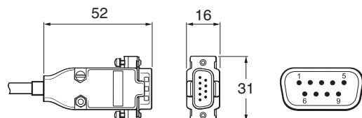
9-pol. SUB-D Stecker
